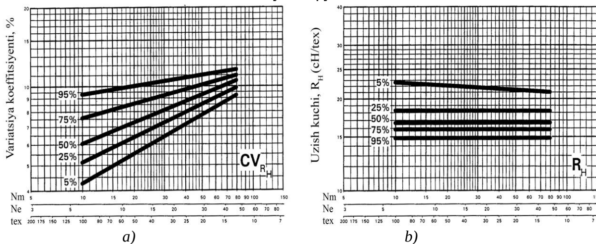
1-rasm. a) ipining pishishligi bo'yicha notekisligi, b) ipining nisbiy pishishligi
